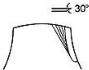
Рис. 19 Заточка ножа
