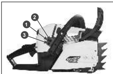
Рис. 20 Винты регулировки карбюратора
