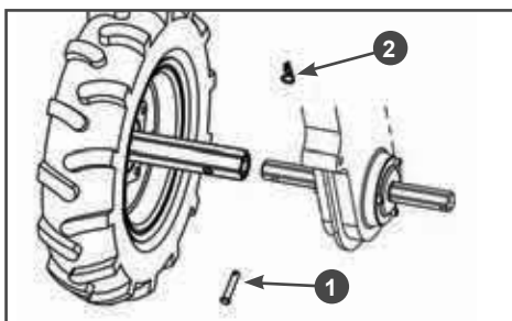
Рис. 6 Установка колес
