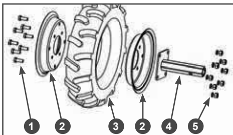
Рис. 5 Сборка колеса
